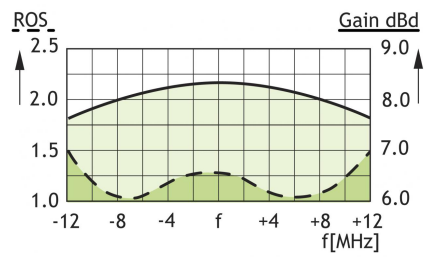
COURBES DE GAIN ET ROS TYPIQUE
